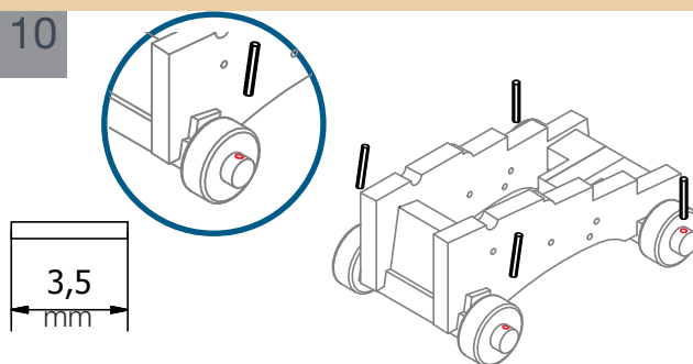
Vista anteriore dell'affusto
