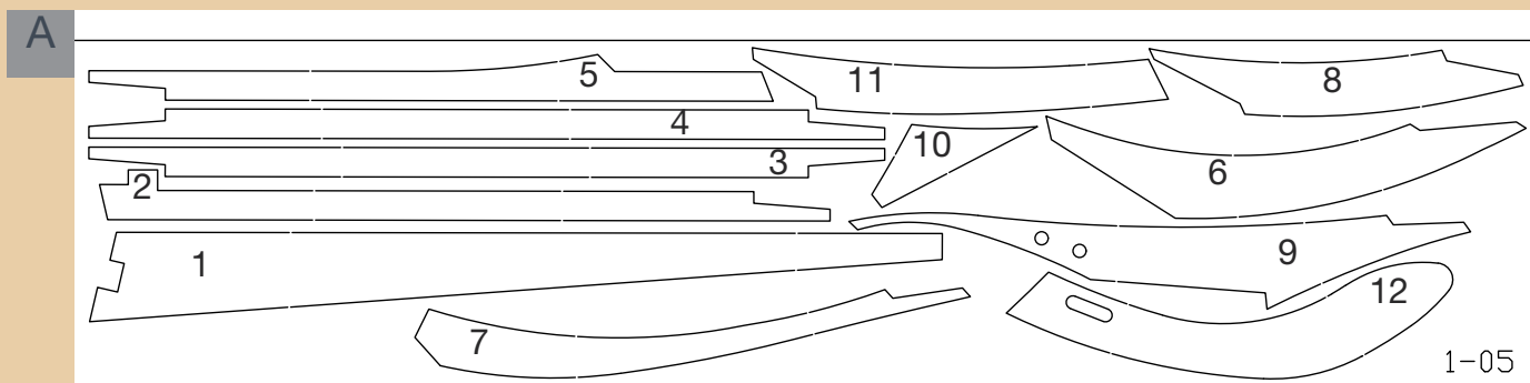
A Componenti della tavoletta 1-05.
