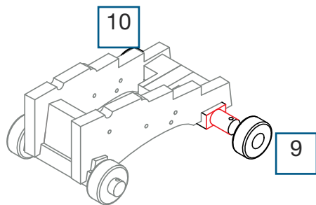
Vista anteriore dell'affusto
