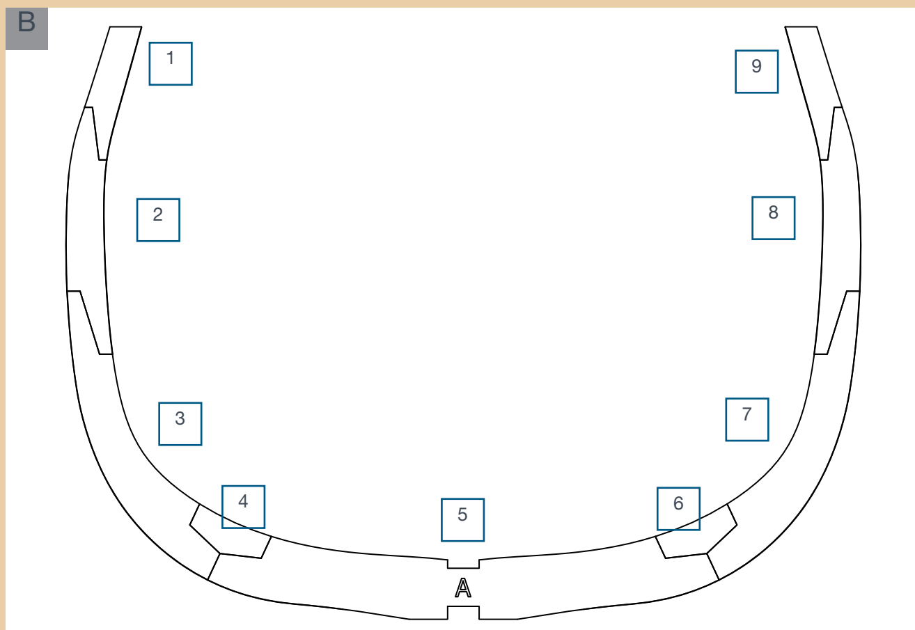
B Stampate questo disegno (Set 01) su un foglio A4 in scala 1:1. Nella figura sono riportati i numeri dei pezzi della tavoletta 1-02. La numerazione dei pezzi corrisponde all'ordine con cui devono essere montati.
