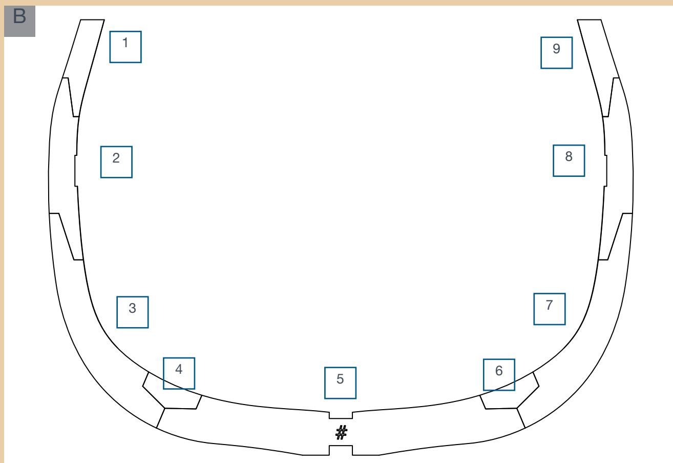
B Stampate questo disegno (Set 01) su un foglio A4 in scala 1:1. Nella figura sono riportati i numeri dei pezzi della tavoletta 1-01. La numerazione dei pezzi corrisponde all'ordine con cui devono essere montati.
