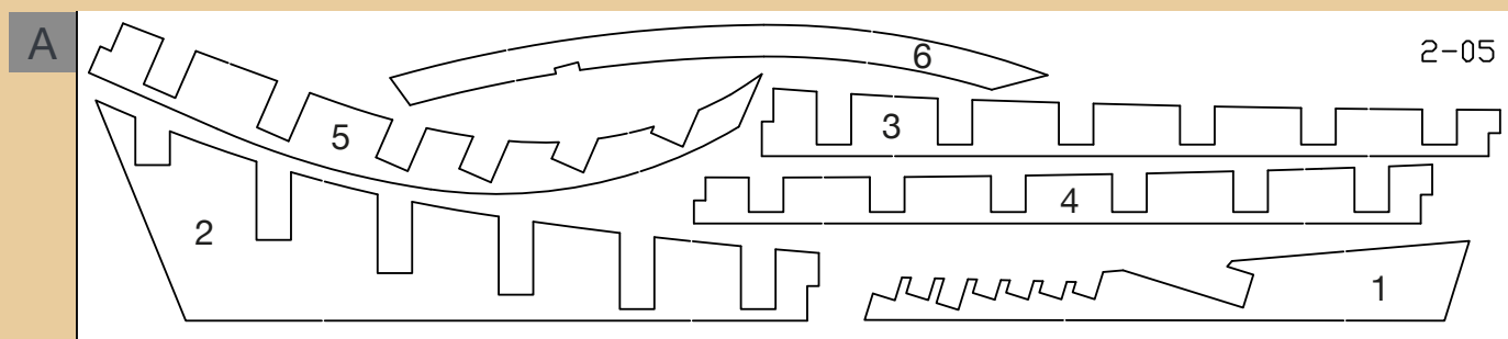
A Componenti della tavoletta 2-05.
