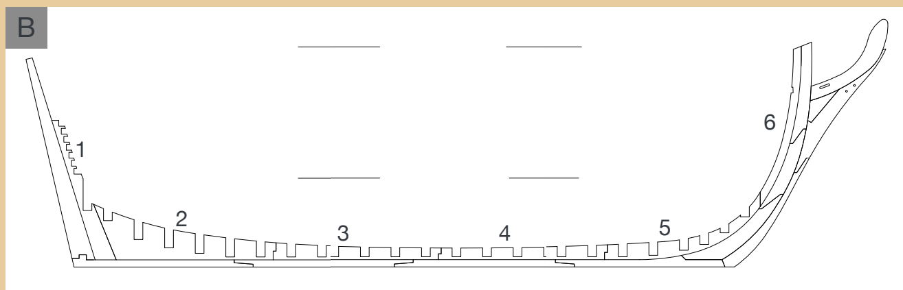
B Questo è il disegno della chiglia completata con le sedi per le ordinate.
