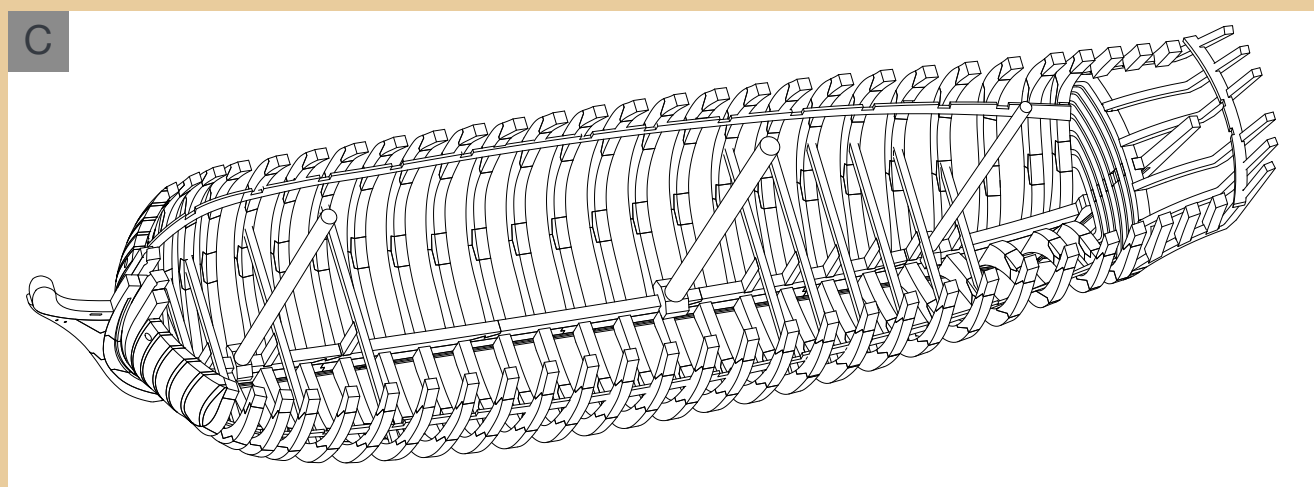
C La figura mostra la struttura dello scafo con le basi delle ordinate che si incastrano nella chiglia.
